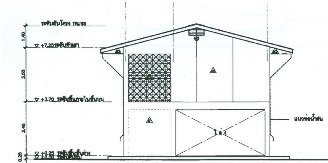
รูปด้าน ② NTS.
