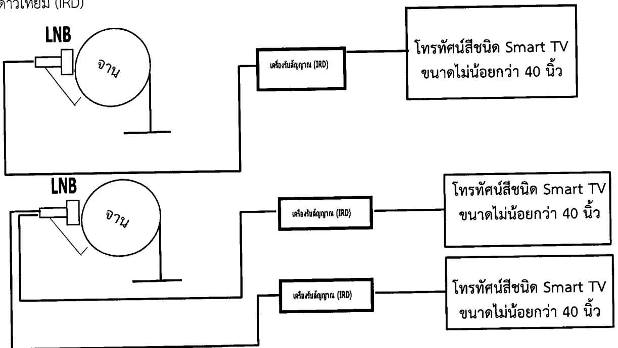
ภาพประกอบการติดตั้งจานดาวเทียม กลุ่มที่ 2
